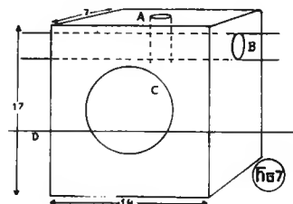
Diagram van het werkstukje, waaruit de draadslede moet groeien A = gat voor ter bevestiging op as dienende schroef B = boorgat voor as C = 10 m.M. diameter voorzien van met transport-as corresponderende draad D = geeft aan op welke hoogte het blokje moet worden afgeznagd. De lijn is door den teekenaar iets te laag gesteld
