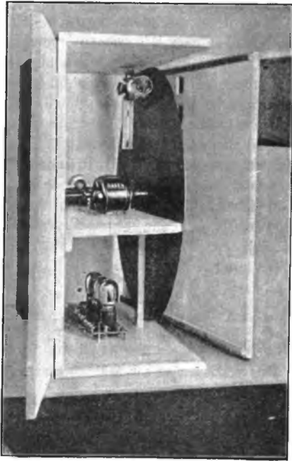
Binnen-aanzicht van den Daven radio-visie-ontvanger.
