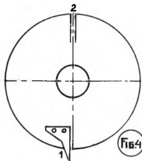
Flens, voorzien van aanslagnok (1) en zaagsnede (2)
