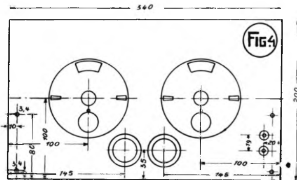
De frontplaat van de Kortegolf-ontvanger, schaal 1 : 4.
