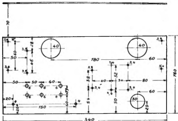
Fig 5. Boorplan van den grondplaat der K.G. Ontvanger van onderen gezien. Schaal 1:4.
