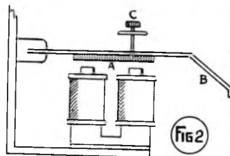
Rem-magneet, waarin A = anker B = omgebogen klepel-arm C = contact-schroef, thans instel-inrichting
