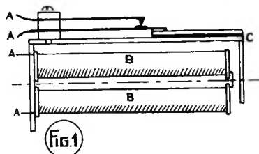
Relais, volgens normaal in den telefoondienst gebruikelijk model
